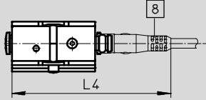
SDE5-...-M8, plug version
